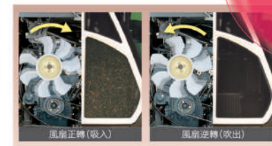
散熱器，去除防塵網的塵埃 逆轉風扇
